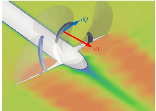
图2 螺旋桨叶元体
