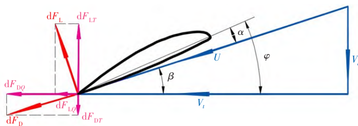
图 1 叶素动量理论
