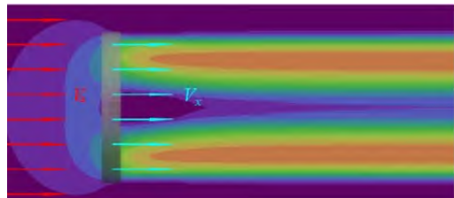
图4 基于真实螺旋桨载荷分布的诱导速度场
