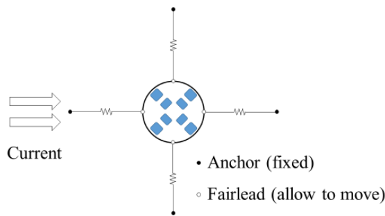
图 1 数值模拟中的系泊系统示意图
