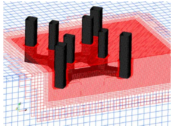
图 4 重叠网格局部图
