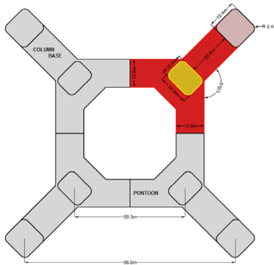
图 2 平台俯视图 [15]
