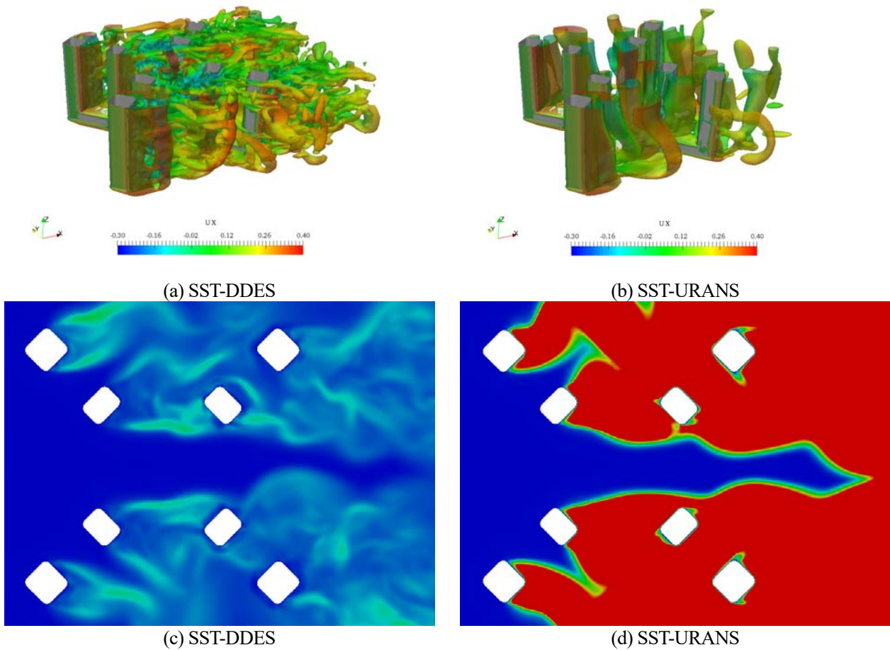
图 5 SST-DDES 和 SST-URANS 得到的(a), (b)涡量图和(c), (d) z=-0.5m 处的湍流粘度
