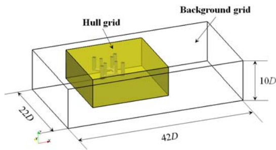
图 3 计算域和嵌套网格
