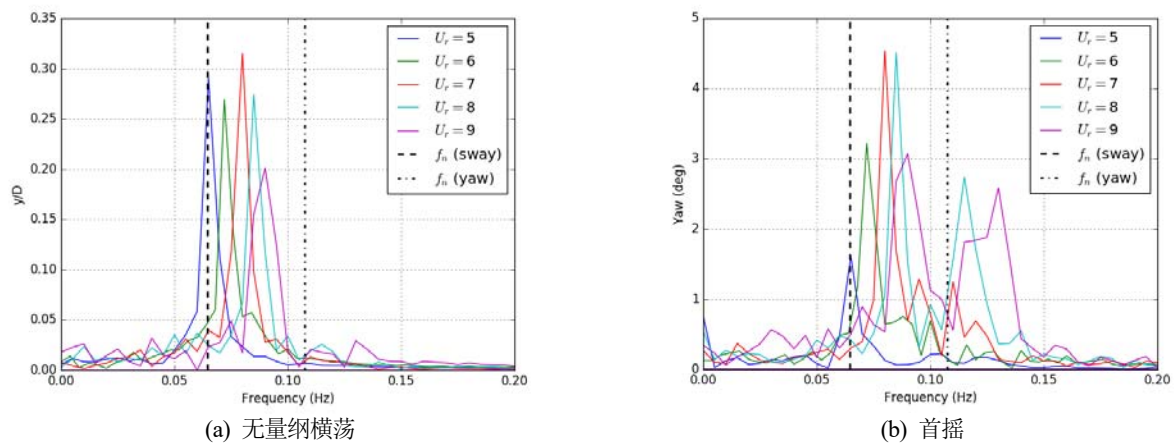
图 9 横荡和首摇响应的快速傅里叶变换
