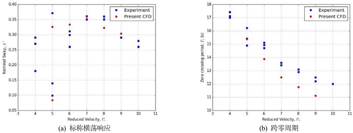
图 8 不同折合速度下的标称横荡响应和跨零周期
