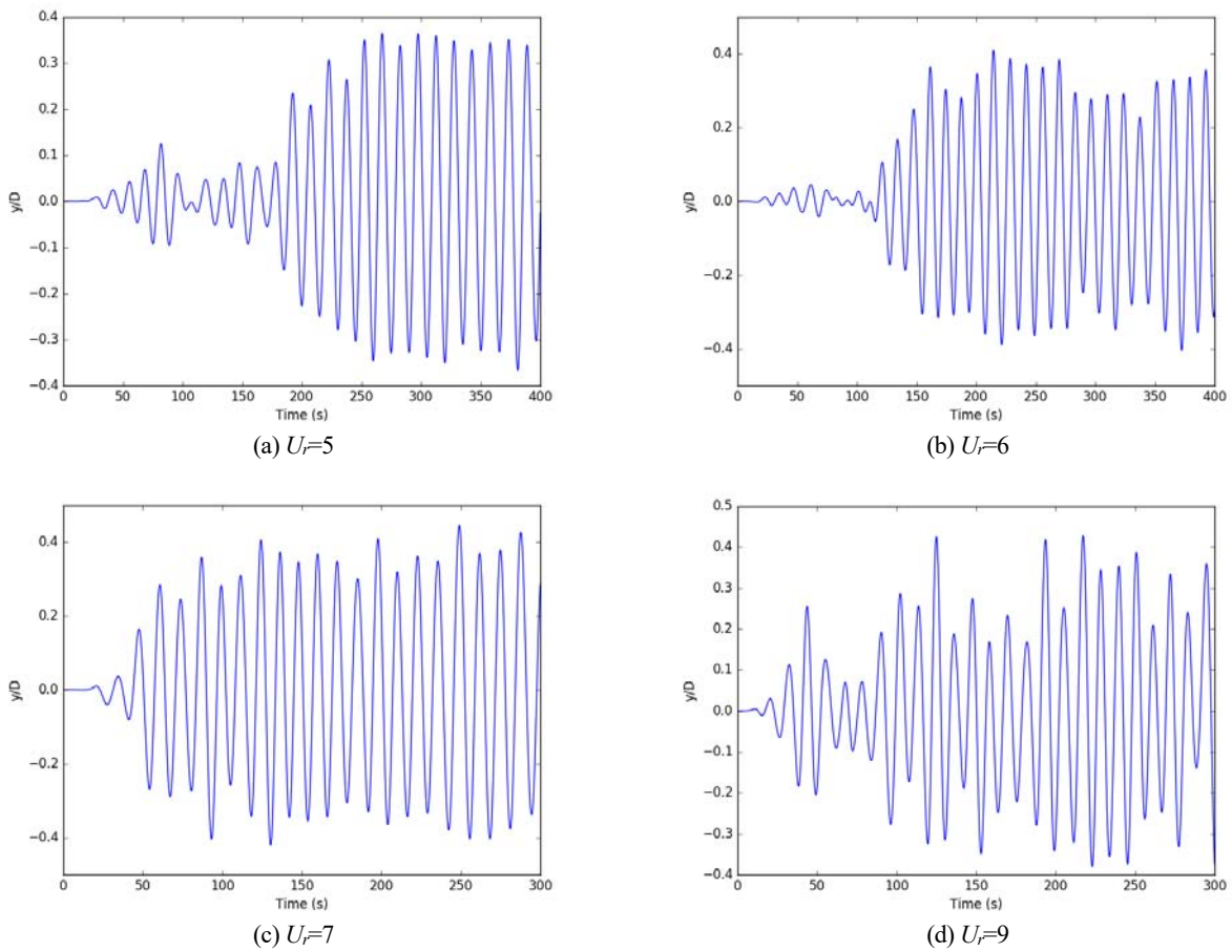
图 7 不同折合速度下的横荡时历曲线
