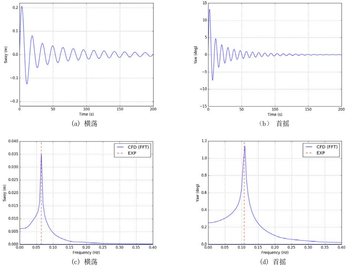
图6 自由衰减的(a), (b)时历曲线和(c), (d)快速傅里叶变换频谱分析
